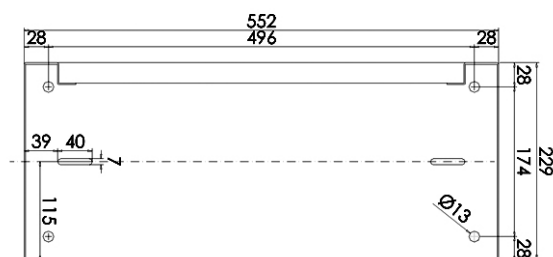
Bovenaanzicht
