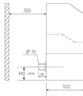
Zijaanzicht
