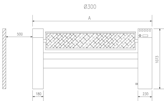
Vooraanzicht
